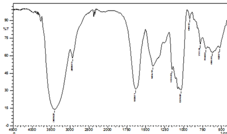
Gambar 7. Spektrum FTIR scleroglucan pada media PDB menggunakan substrat gula cair 7%
