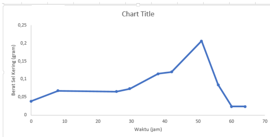
Gambar 3. Kurva pertumbuhan S.rolfsii pada PDB
