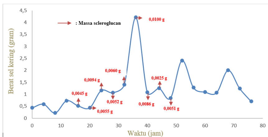
Gambar 5. Kurva produksi scleroglucan pada PDB dengan substrat gula cair 7%
