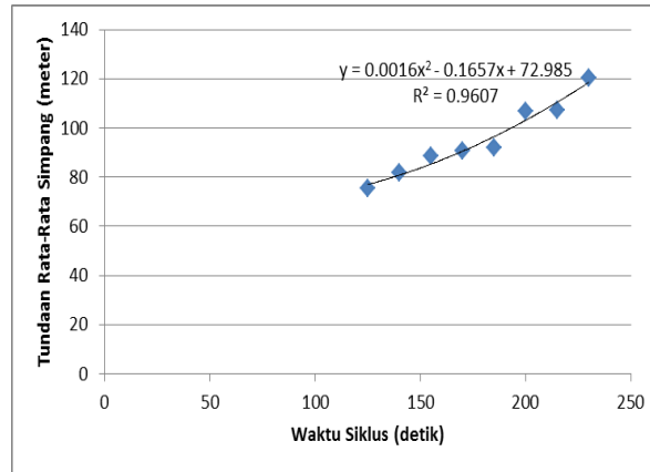
Gambar 8. Tundaan Rata-Rata untuk Simpang vs Waktu Siklus
