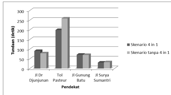
Gambar 6. Perbedaan Tundaan antara Kondisi “4 in 1” dan Tanpa “4 in 1”
