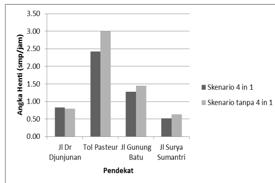
Gambar 7. Perbedaan Angka Henti antara Kondisi “4 in 1” dan Tanpa “4 in 1”
