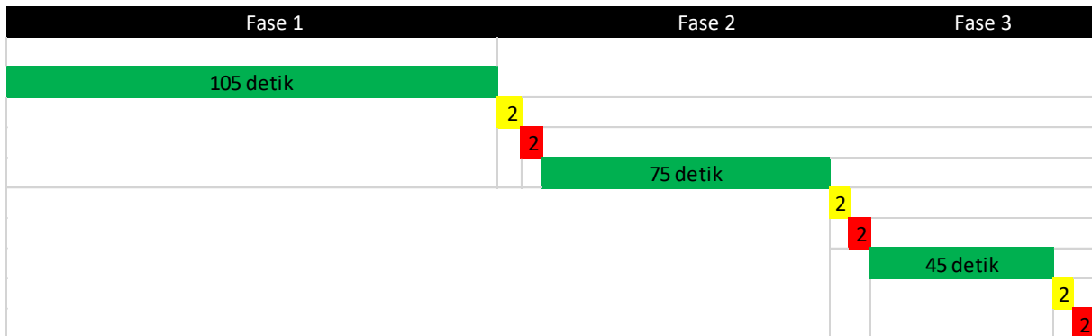
Gambar 4. Waktu operasi sinyal lalu lintas per fase
