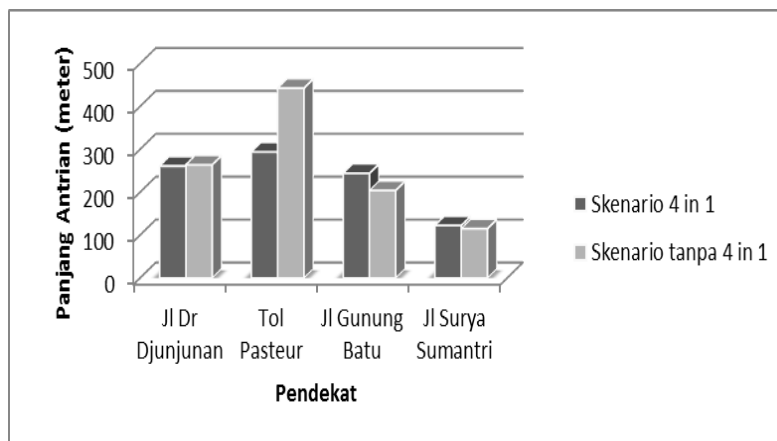
Gambar 5. Perbedaan Panjang Antrian Antara Kondisi “4 in 1” dan Tanpa “4 in 1”
