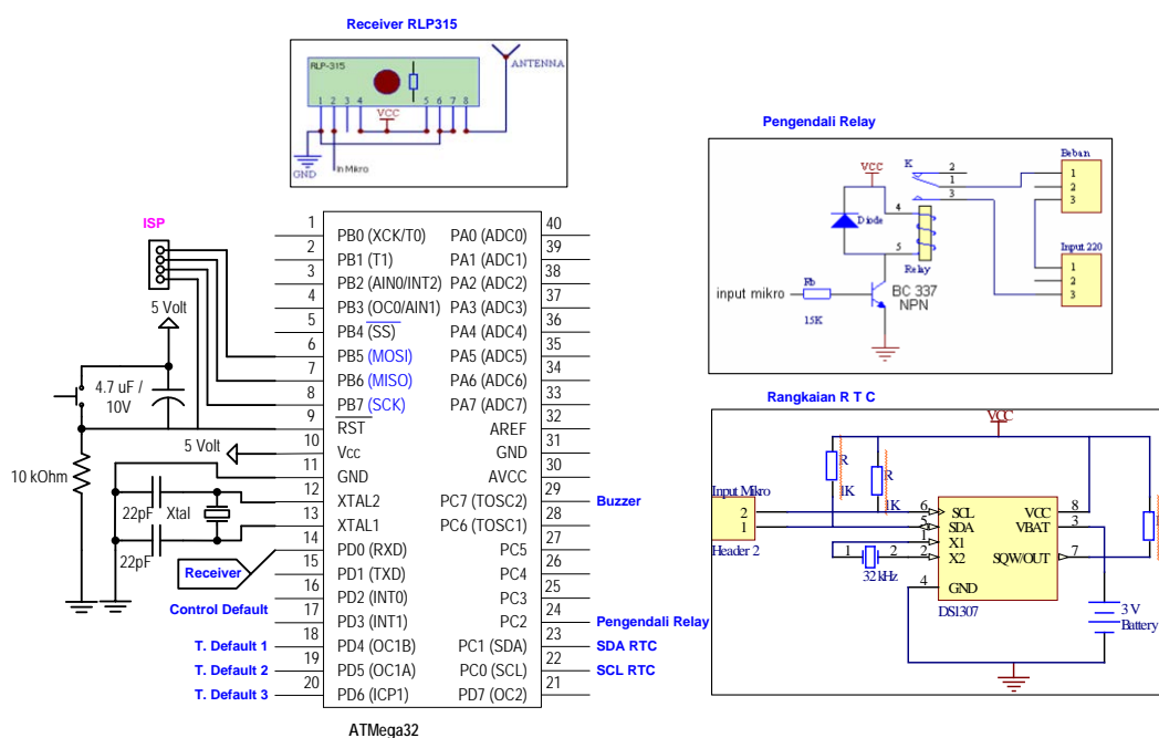
Gambar 3. Skema diagram sistem ATS
