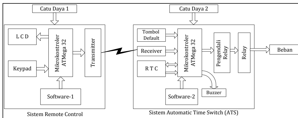
Gambar 1. Diagram blok sistem ATS-C2I versi 2
