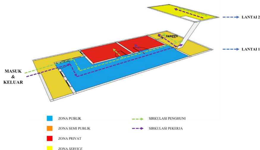
Gambar 7. Zoning dan Pola Sirkulasi Rumah Industri Rajut Pak Yusin
