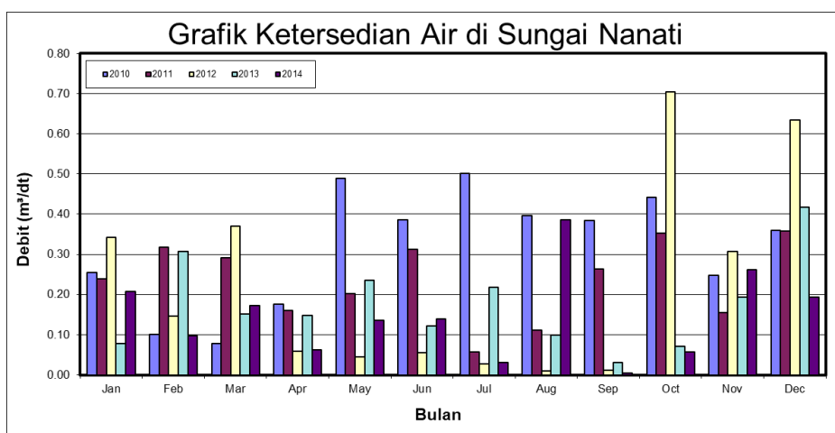
Gambar 1. Grafik ketersediaan air di Sungai Nanati
