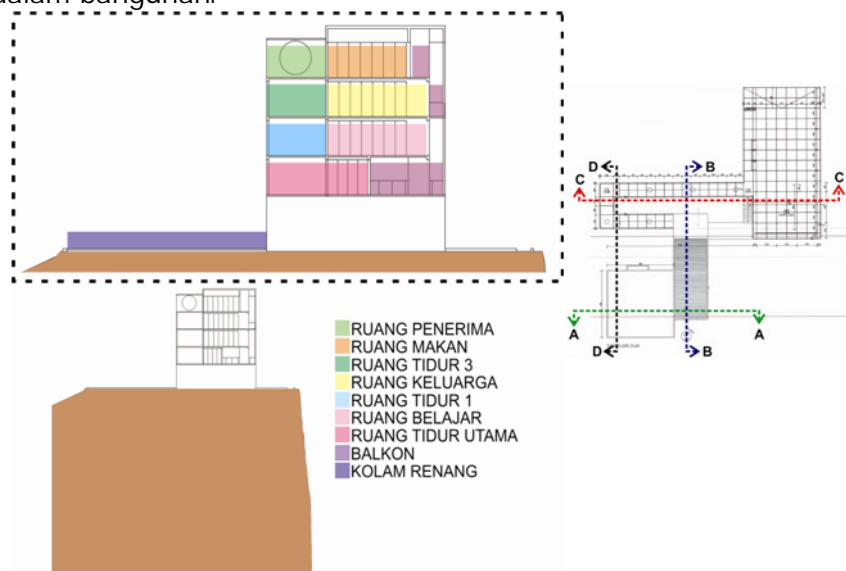
Gambar 7 : Potongan A – A (Sumber: Pramestha, 2014, diolah)
