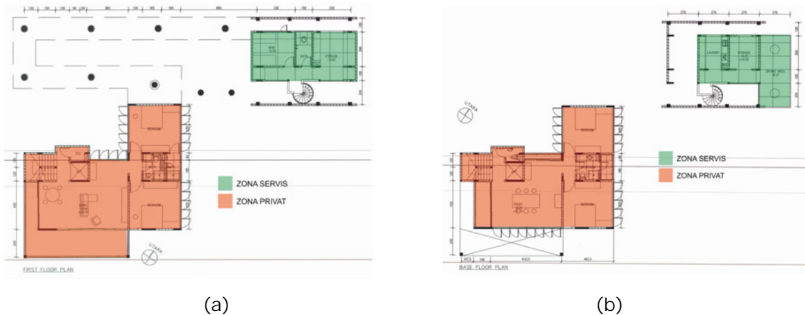
Gambar 5 : a) denah lantai tiga(Sumber : Pramestha, 2014, diolah) dan b) denah lantai dua(Sumber : Pramestha, 2014, diolah)
