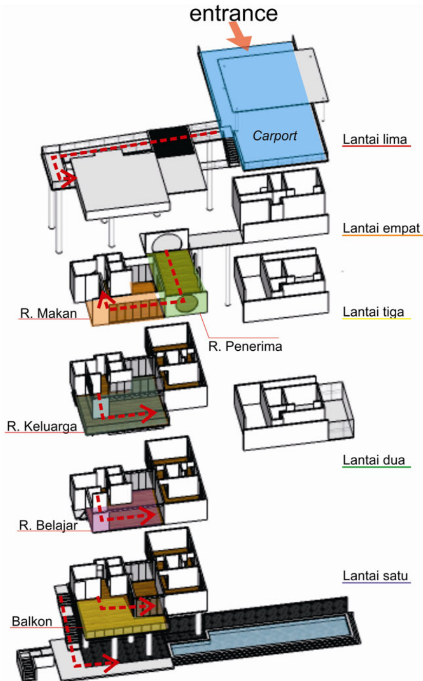
Gambar 11 : Aksonometri (Sumber: Pribadi, 2014)
