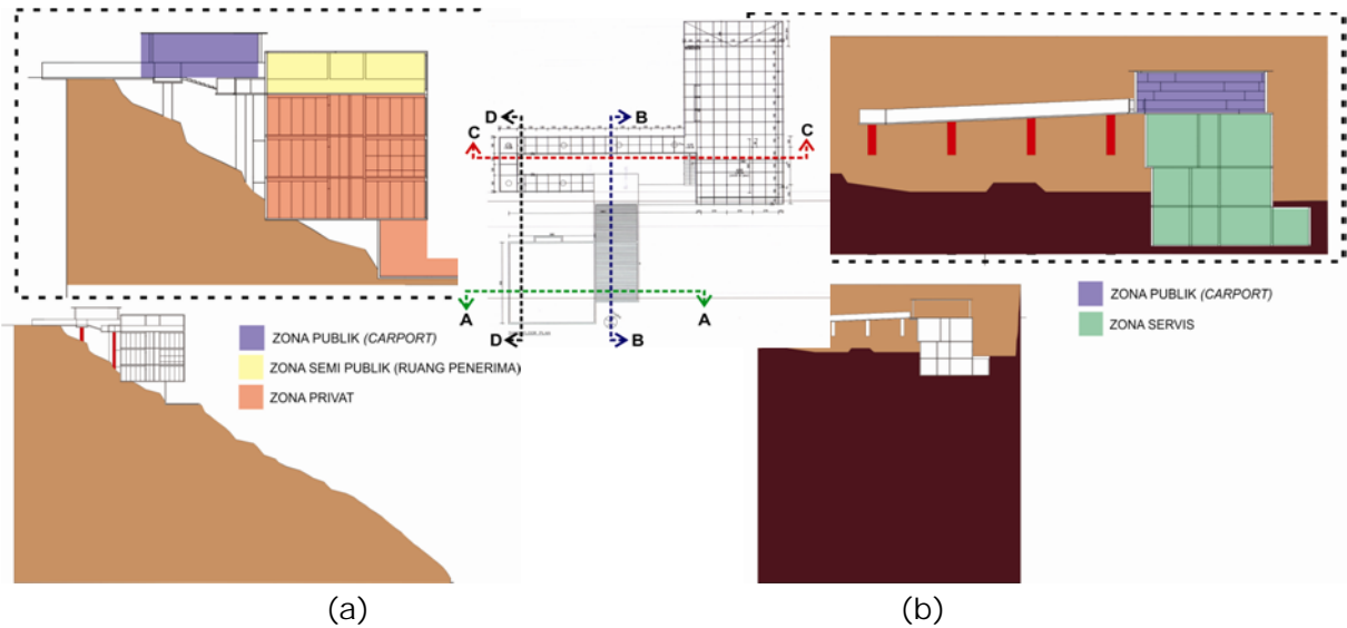
Gambar 6 a) Potongan B – B (Sumber : Pramestha, 2014, diolah dan b) Potongan C – C (Sumber : Pramestha, 2014, diolah
