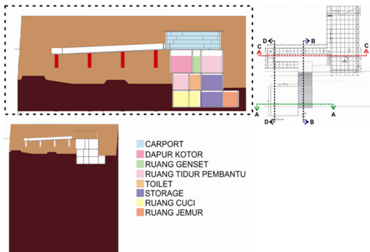
Gambar 9 : Potongan C – C (Sumber: Pramestha, 2014, diolah)
