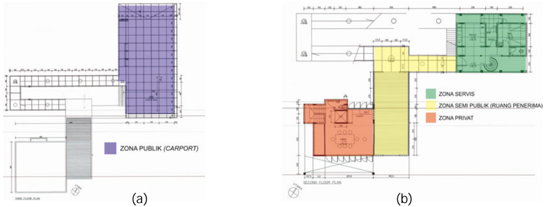
Gambar 4 : a) denah lantai lima(Sumber : Pramestha, 2014, diolah) dan b) denah lantai empat(Sumber : Pramestha, 2014, diolah)
