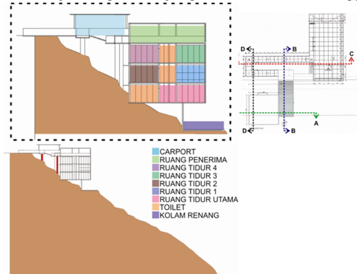
Gambar 8 : Potongan B – B (Sumber: Pramestha, 2014, diolah)
