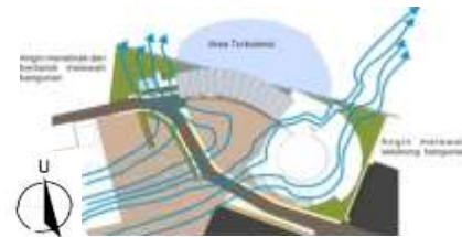
Gambar 18. Orientasi bangunan terhadap arah angin.
