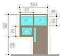
Gambar 26. Desain bukaan tipe 1a.
