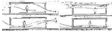
Gambar 10. Perbedaan lokasi bukaan akan mempengaruhi pola pergerakan udara dalam ruang.
