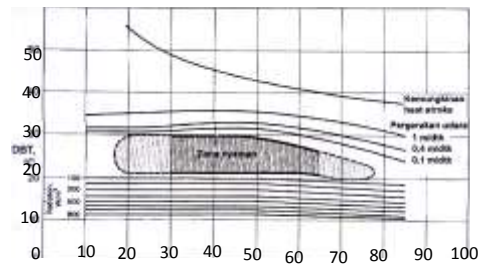
Gambar 13. Diagram kenyamanan termal Sumber: Satwiko, Prasasto, 2004, Fisika Bangunan 1.
