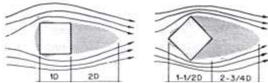
Gambar 4. Orientasi bangunan persegi terhadap arah angin.
