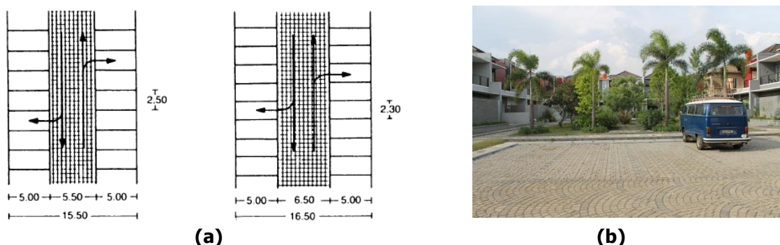
Gambar 3. (a) Layout parkir standart, (b) Area parkir bersama perumahan the mansioan ( Sumber : Neuvart Data Arsitek Jilid 1, data hasil survey lapangan )
