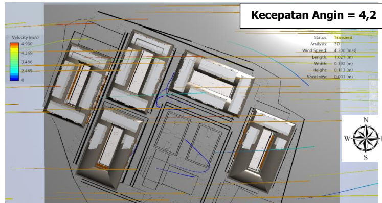
Gambar 6. Blok Rusun Cingised Terhadap Sirkulasi Pergerakan Angin (Sumber: Hasil Analisis Flow Design,2015)
