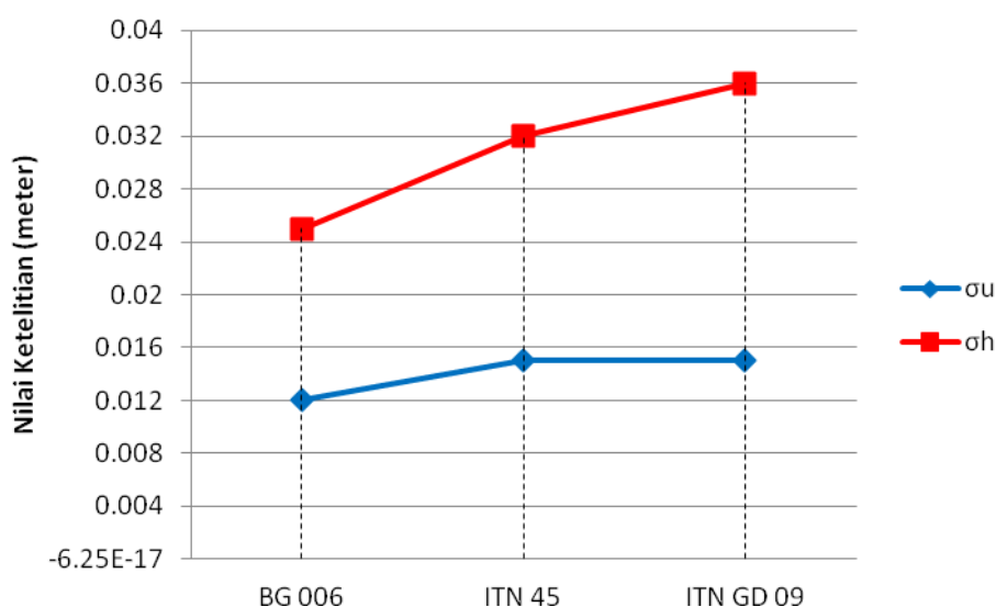
Gambar 2. Grafik Ketelitian Posisi Titik
