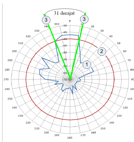
Gambar 14. Pola Radiasi dan Beamwidth Reflector Wajan
