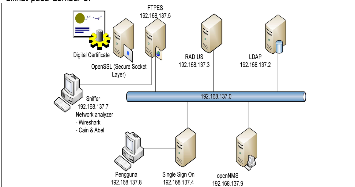
Gambar 5. Struktur dan Topologi
