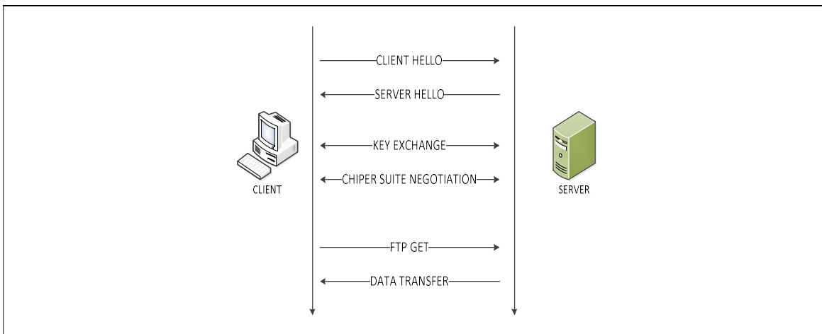
Gambar 10. Mekanisme SSL
