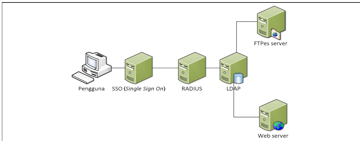
Gambar 9. Mekanisme SSO
