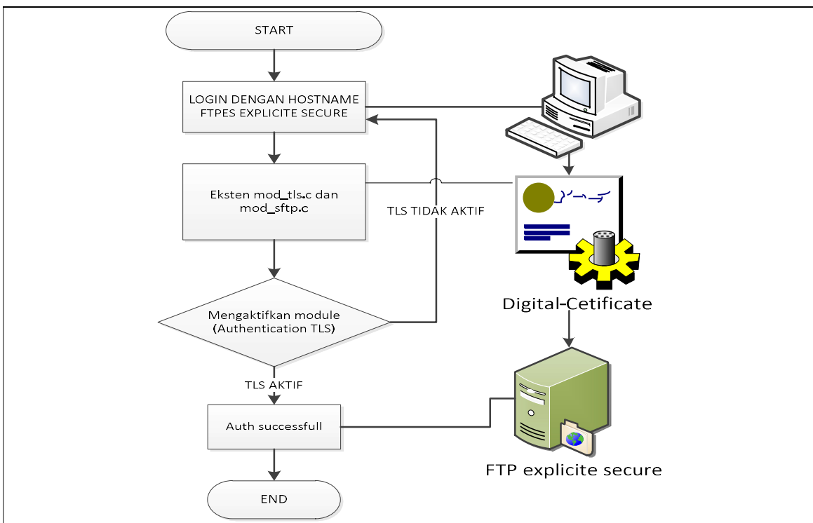
Gambar 11. Mekanisme Explicite FTPS
