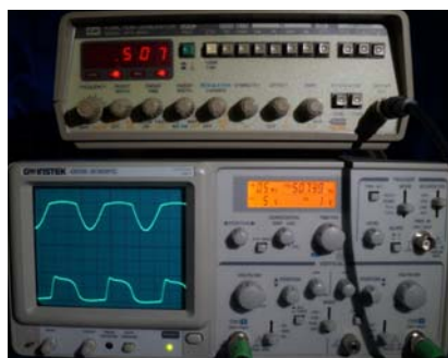
Gambar 9. Bentuk sinyal dengan input frekuensi 500 Hz
