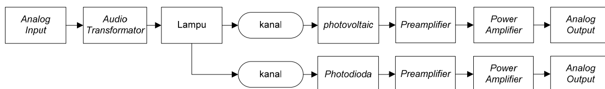
Gambar 2. Blok Diagram Sistem.
