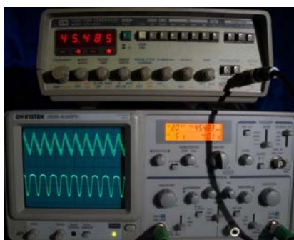
Gambar 12. Bentuk sinyal dengan input frekuensi 45,485 kHz
