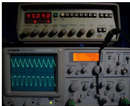
Gambar 11. Bentuk sinyal dengan input frekuensi 45 kHz
