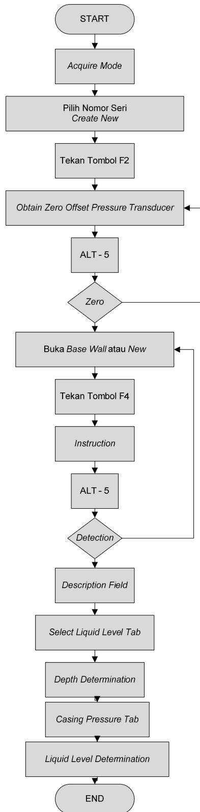
Gambar 3. Flowchart Langkah-langkah Dasar untuk Pengukuran Liquid Level
