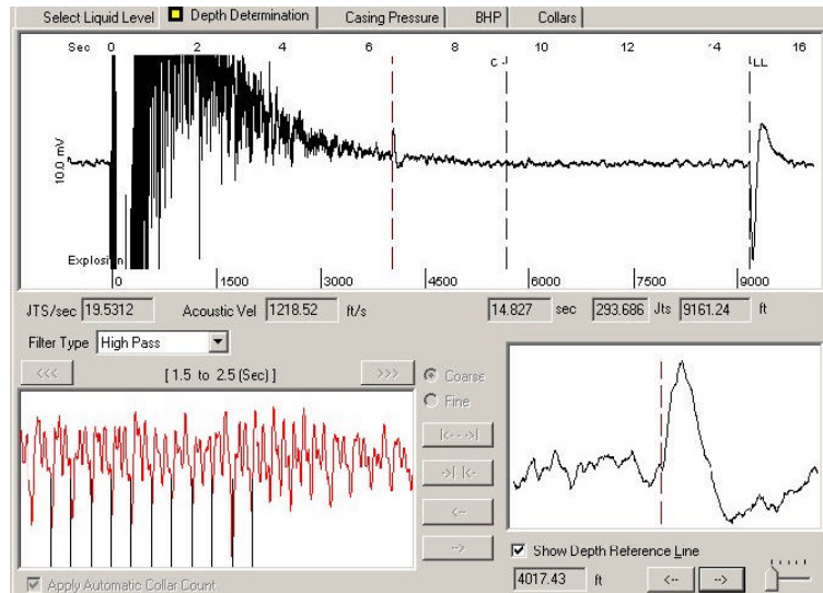
Gambar 5. Bentuk denyut acoustic dari chamber remote fire gas gun
