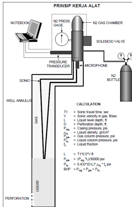
Gambar 2. Peralatan dan prinsip kerja peralatan serta perhitungan yang dilakukan untuk mendapatkan tekanan bawah permukaan.
