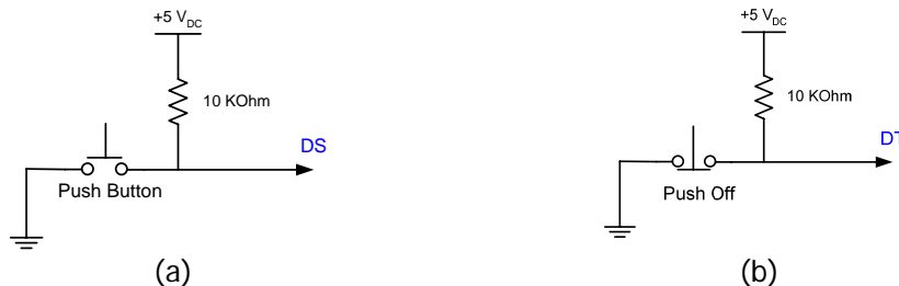
Gambar 4. Realisasi rangkaian (a) saklar pembuka ; (b) sensor pintu
