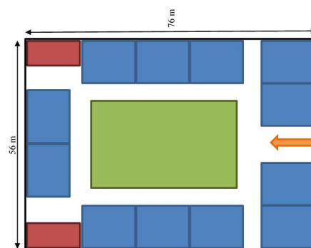
Gambar 5. Sketsa Gedung Pengujian Indoor
