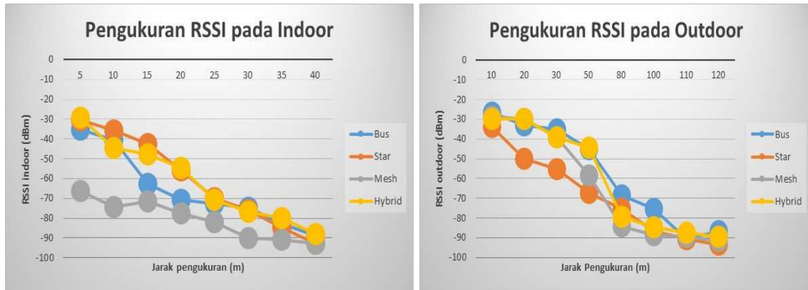
Gambar 7. Grafik Hasil Pengujian RRSI (dBm) pada Kondisi Indoor dan Outdoor
