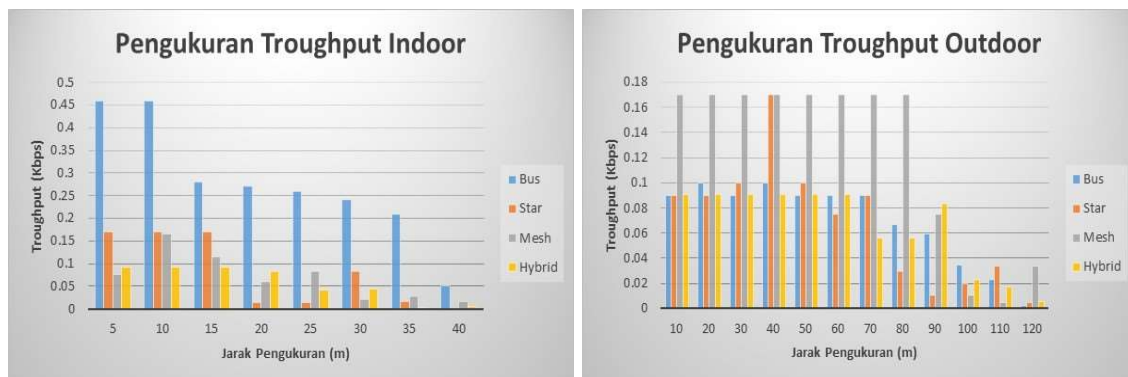
Gambar 8. Grafik Hasil Pengujian Troughput pada Kondisi Indoor dan Outdoor
