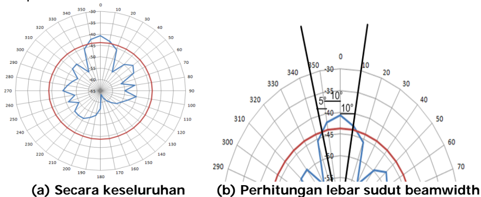
Gambar12. Pola Radiasi dan Beamwidth Verikal
