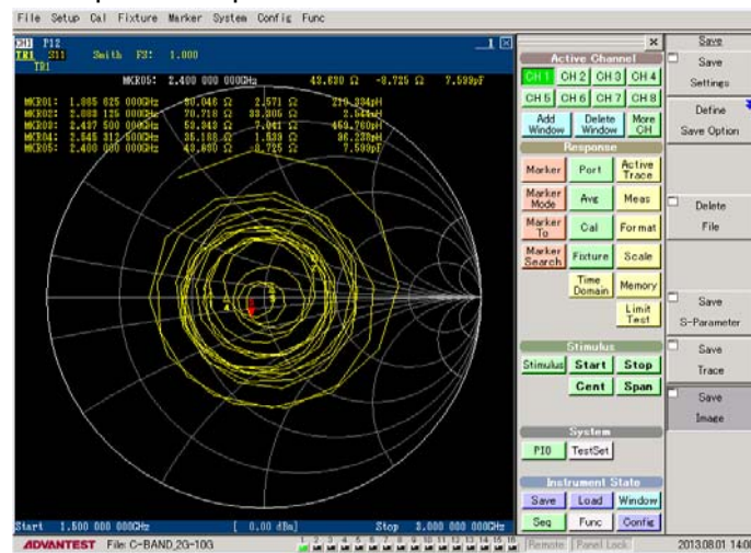
Gambar 10. Hasil pengukuran Impedansi
