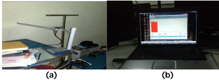
Gambar 15. Pengukuran Aplikasi Antena pada notebook (a) antenna yagi yang diukur (b) notebook yang berfungsi sebagai penerima
