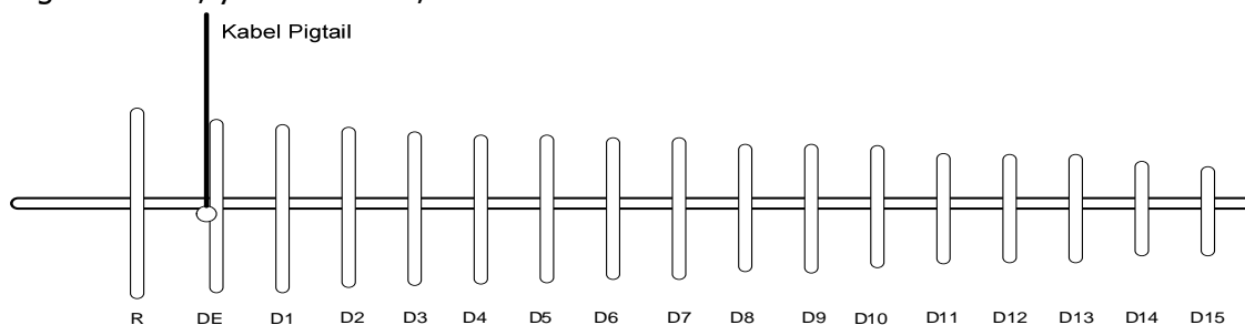
Gambar 1. Pemodelan Antena yagi.
