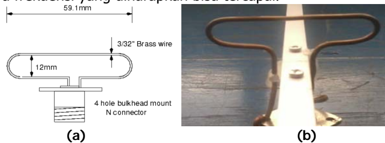
Gambar 5. Skema pemasangan antena dipole (a) gambar skema ukurannya (b) antena folded dipole yang sudah tersambung pada N konektor
