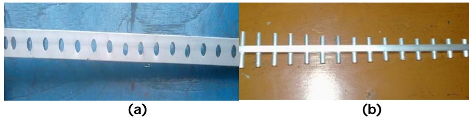
Gambar 3. Pemasangan elemen pada boom (a) boom terbuat dari aluminium (b) elemen yang terpasang pada boom
