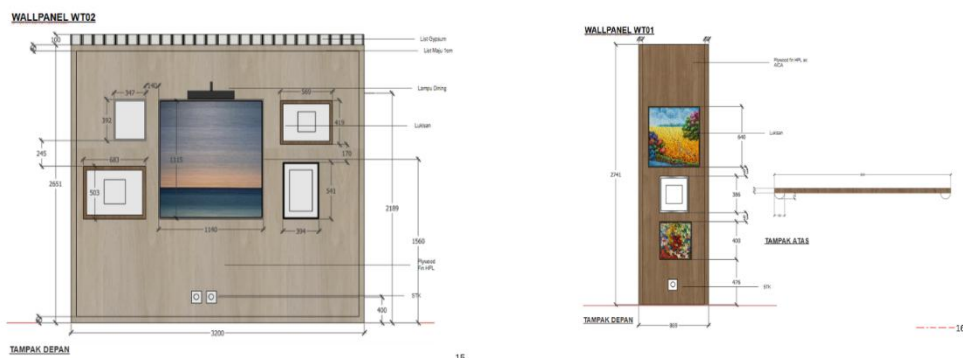
Gambar 5. Tampak dan Potongan Furnitur Living Room Sumber: Arsip BINBO
