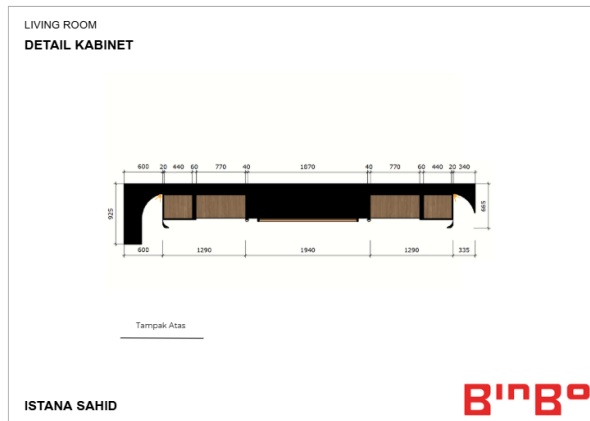
Gambar 3. Tampak Atas Furnitur Living Room Sumber: Arsip BINBO
